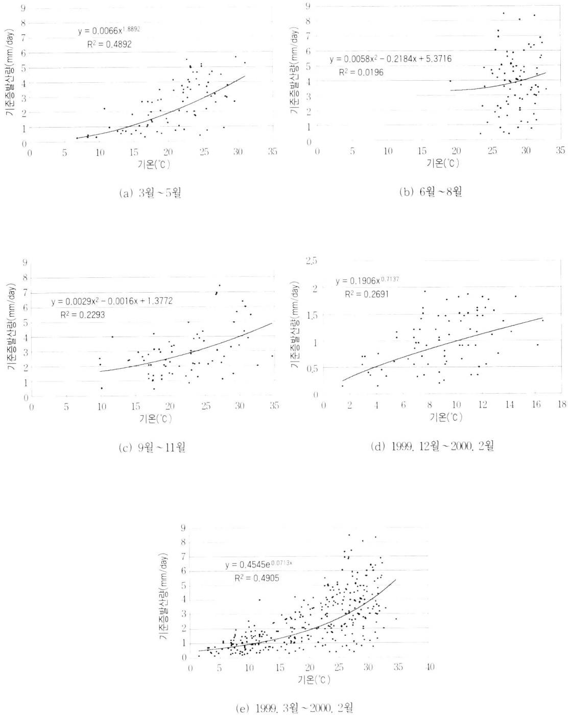
Fig. 4. 기온과 기준작물 증발산량과의 관계
