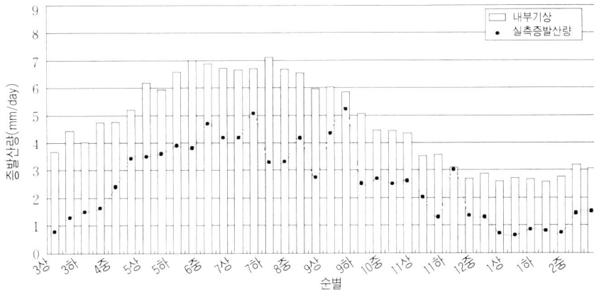
Fig. 9 Blaney-Criddle식과 내부기상을 이용한 추정 순별증발산량
