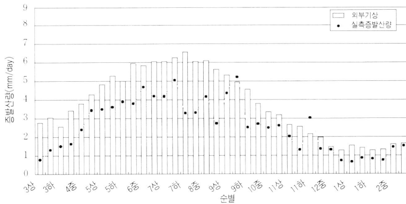
Fig. 10 Blaney-Criddle식과 외부기상을 이용한 추정 순별증발산량
